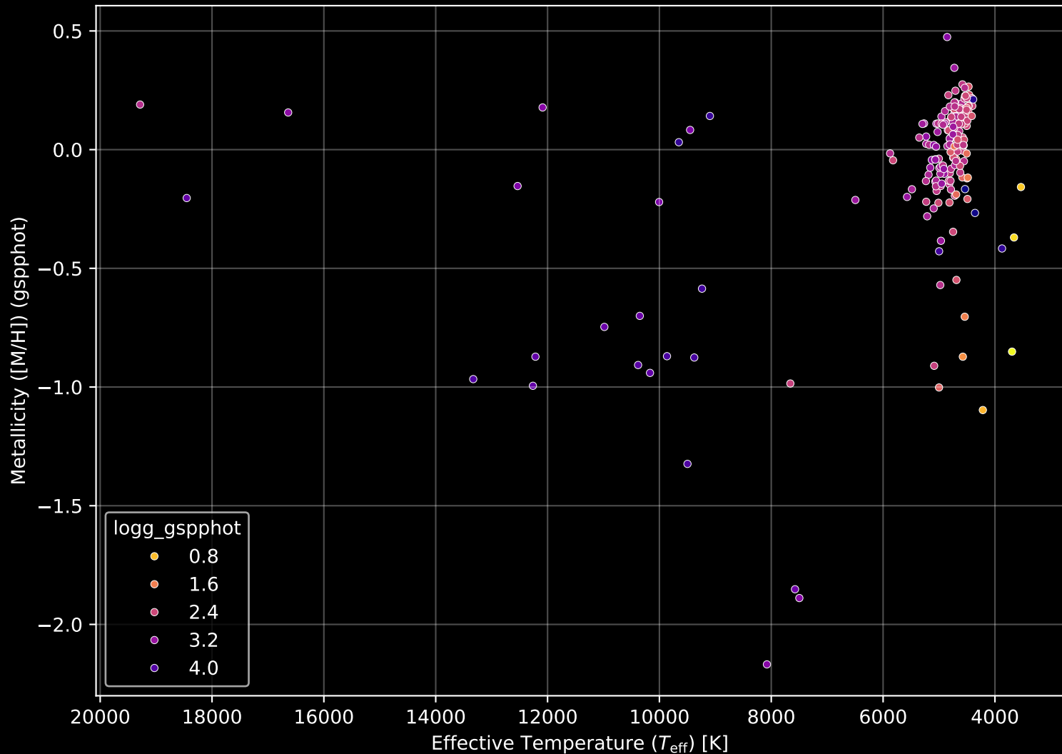
APOGEE DR17 Field: [045+06] Stellar Population Parameters (n= 195)
